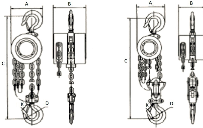
Рис. 1 Основные размеры тали
